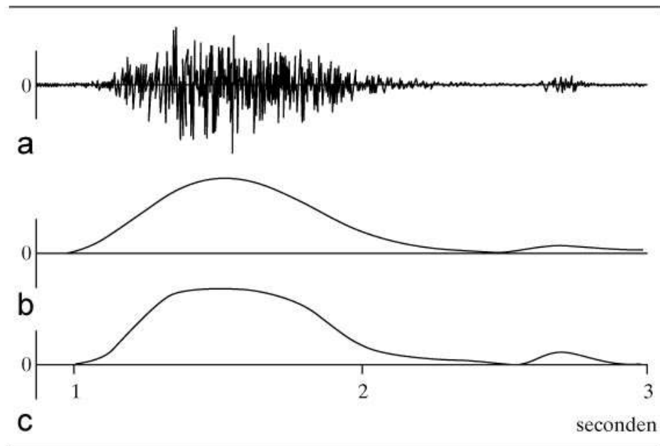
FIGUUR 3. Van het ruwe oppervlakte-elektromyografie(EMG)-signaal (a) bij willekeurig aanspannen kan de omhullende curve bepaald worden (b). Dit zogenaamde 'smoothed rectified' EMG-sig-naal vertoont qua dynamiek grote overeenkomst met de uitgeoefende kracht van de spier (c); op de Y-assen staan arbitraire eenheden.
